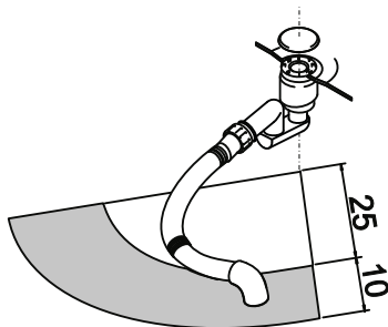
Fig. 6. Abwasserinstallation
