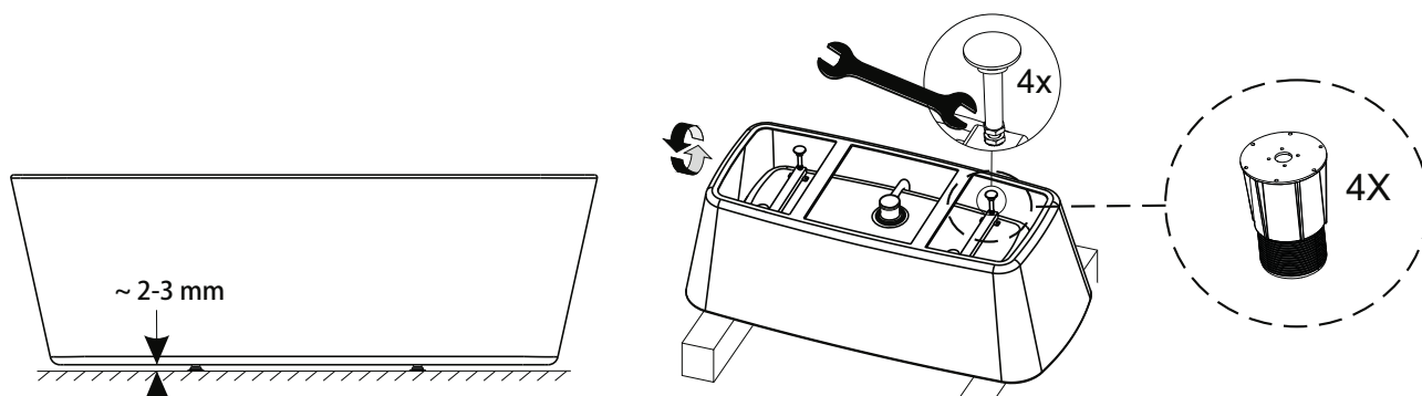
Fig. 2 Patte montage
