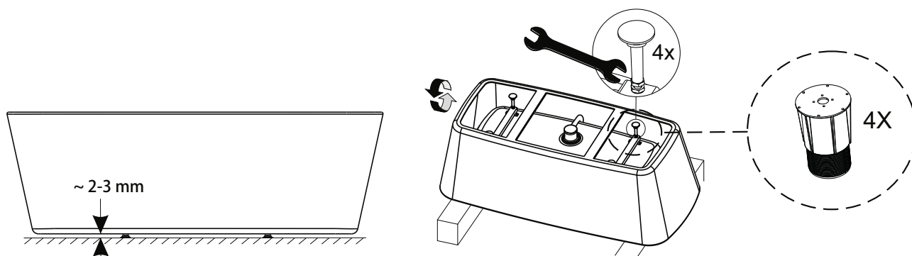
Fig. 2 Poot montage
