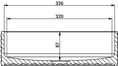
A-A (1 : 3)
