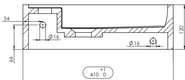
SECTION A-A SCALE 1 : 3
